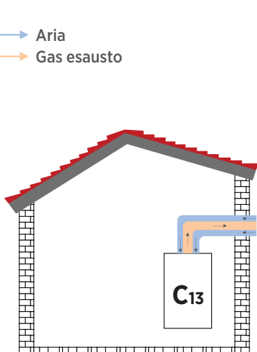
Scarico fumi coassiale
